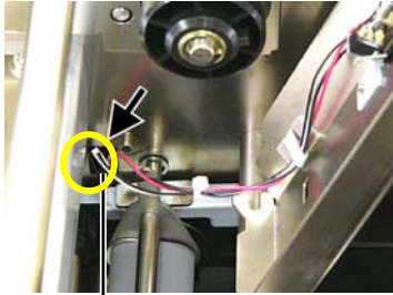
Farbband Ende Sensorkabel
