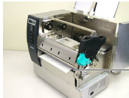
Material Auslass
