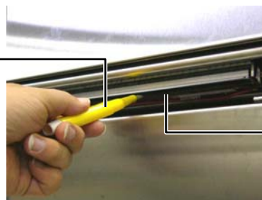
Druckkopf- reinigungsstift
