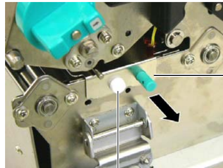
Weiße Handschraube
