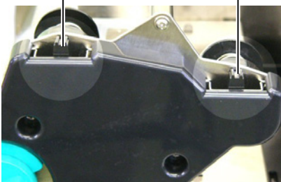
Farbband Justagehebel
